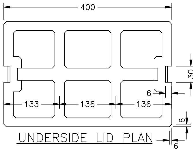
LID PLAN
