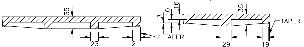
LID SIDE SECTION
