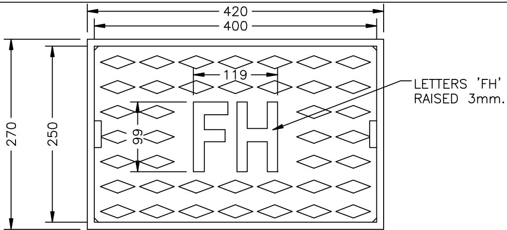
LID PLAN
